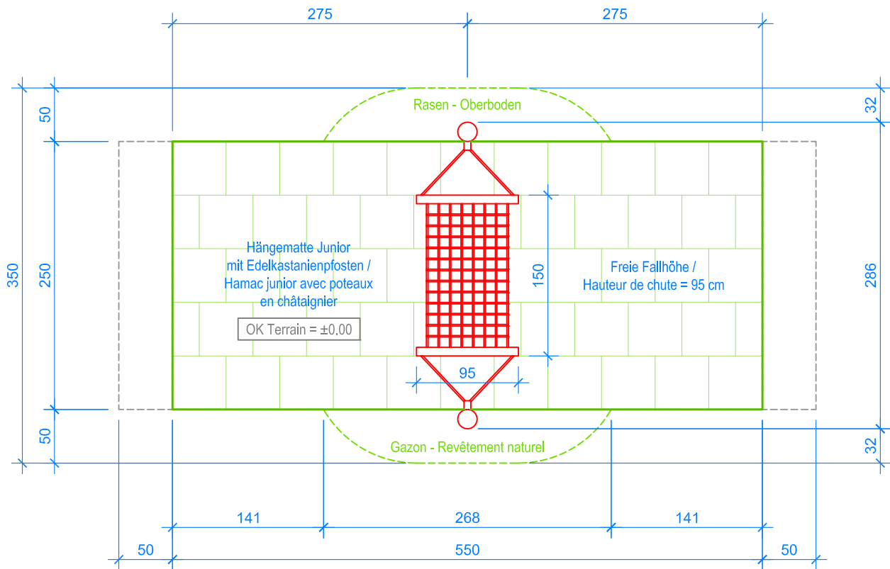
GRUNDRISS / PLAN 1:50
