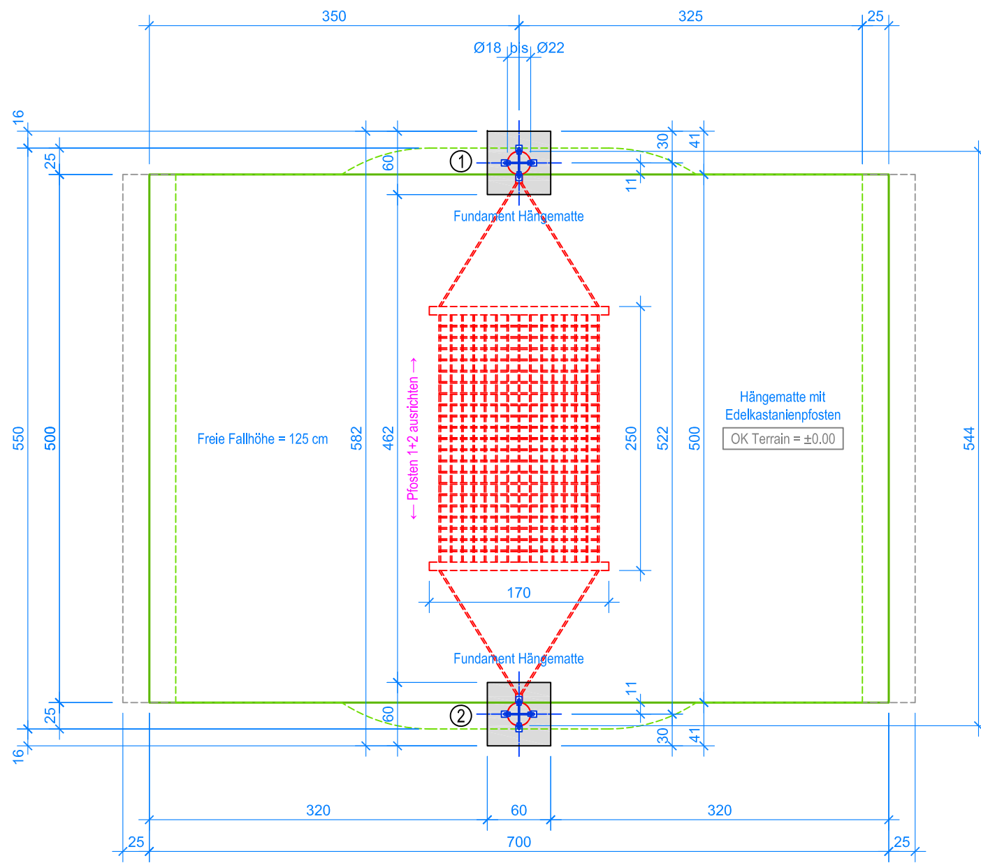
GRUNDRISS 1:50
