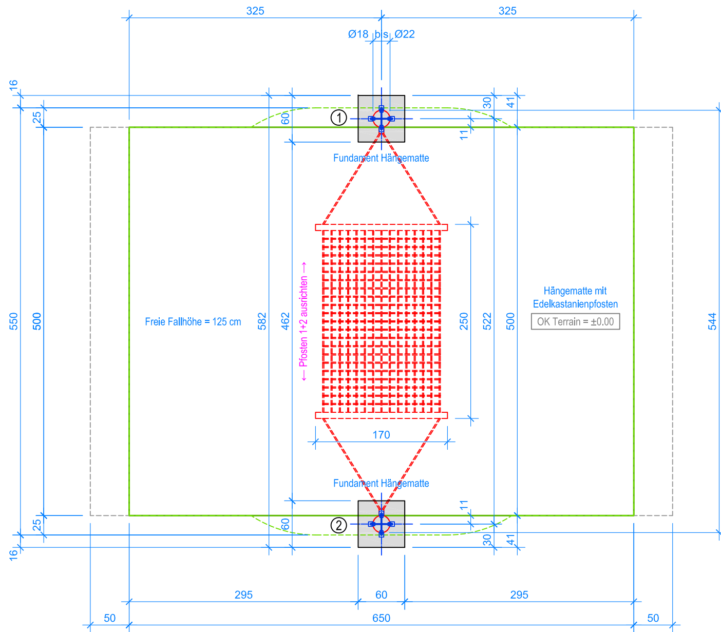
GRUNDRISS 1:50
