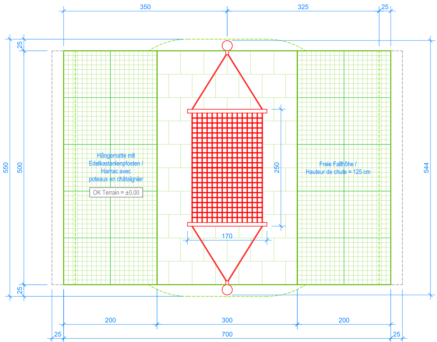
GRUNDRISS / PLAN 1:50
