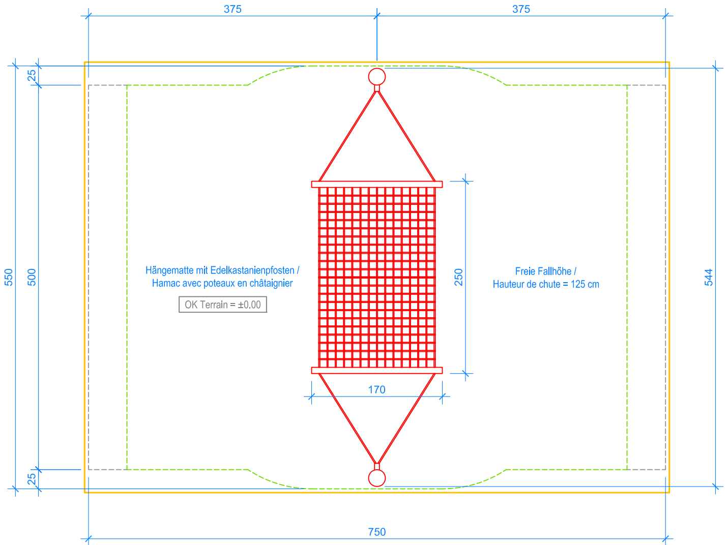
GRUNDRISS / PLAN 1:50
