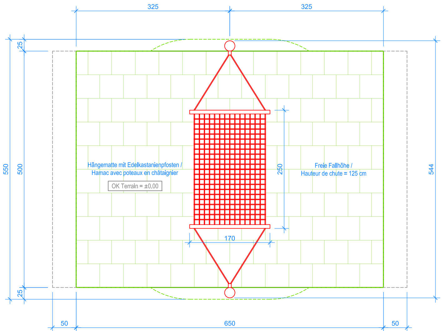
GRUNDRISS / PLAN 1:50
