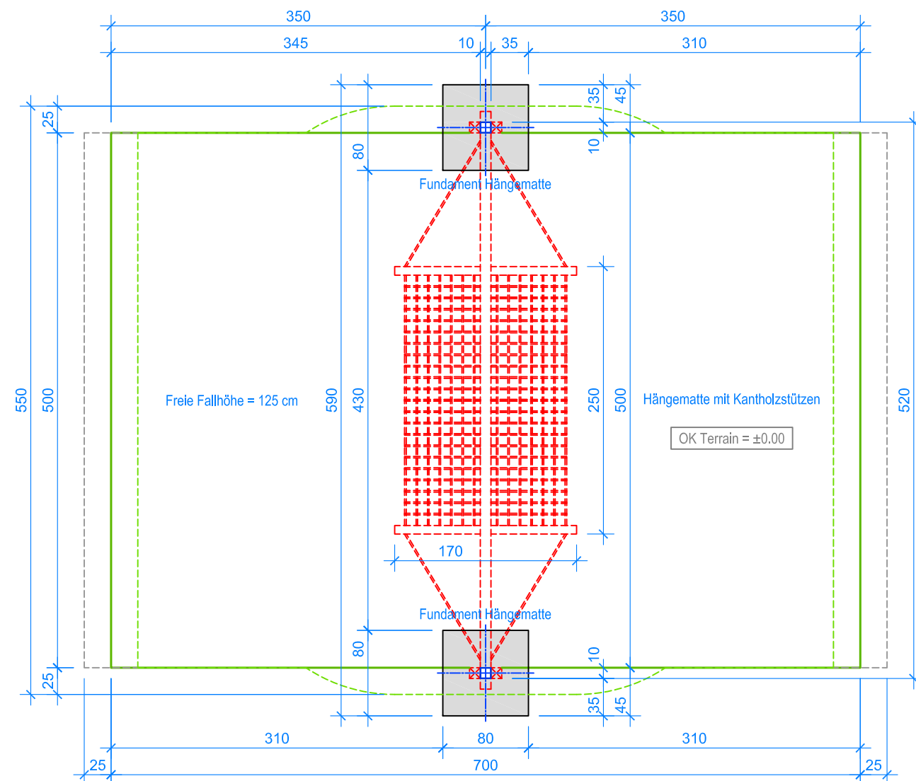
GRUNDRISS 1:50
