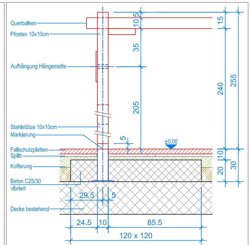
SCHNITT 1:20 FUNDAMENT HÄNGEMATTE
