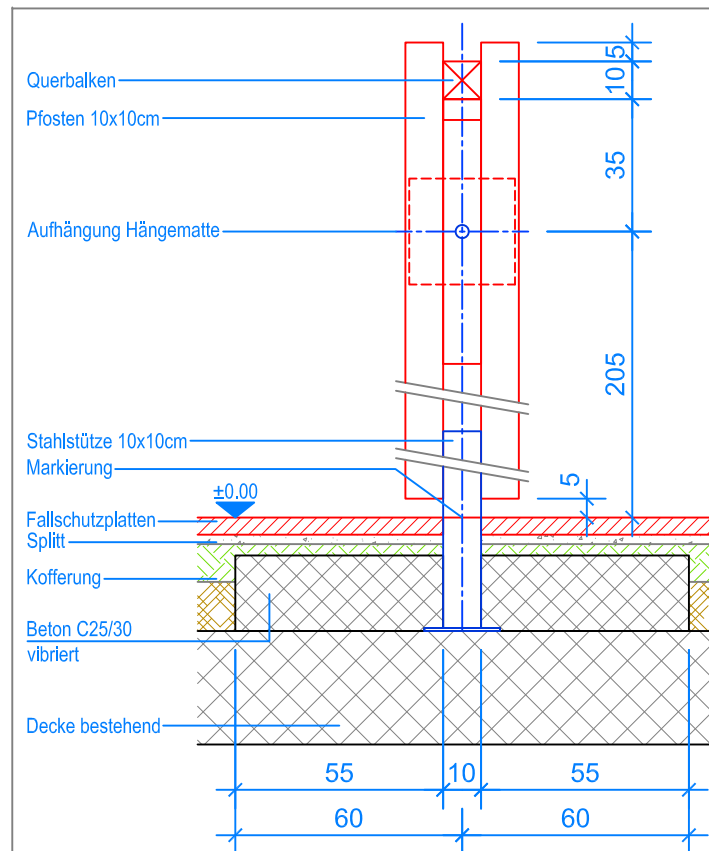
SCHNITT 1:20 FUNDAMENT HÄNGEMATTE
