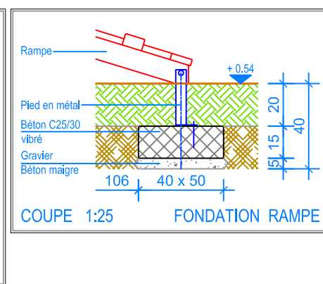
COUPE 1:25 FONDATION ESTRADE
