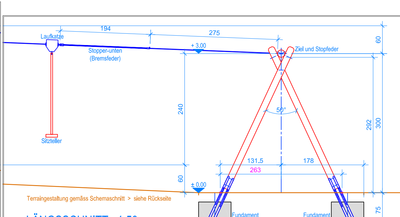
LÄNGSSCHNITT 1:50
