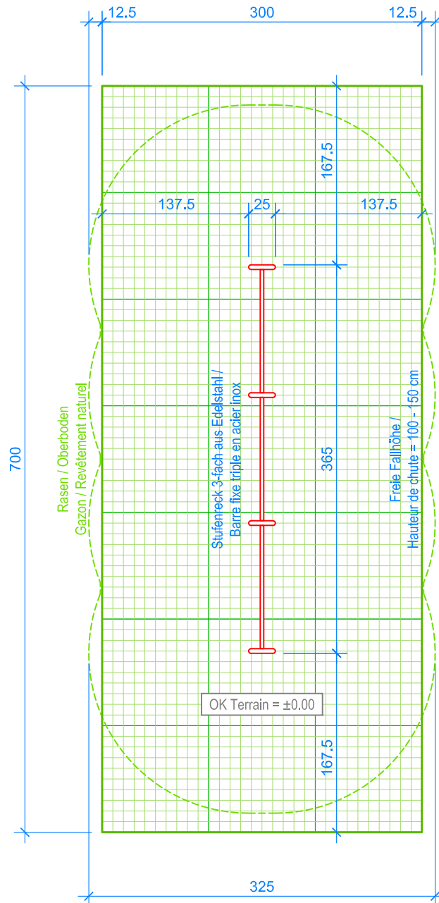
GRUNDRISS / PLAN 1:50
