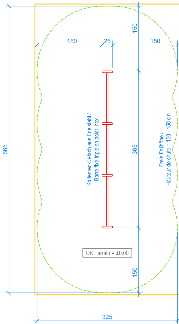
GRUNDRISS / PLAN 1:50
