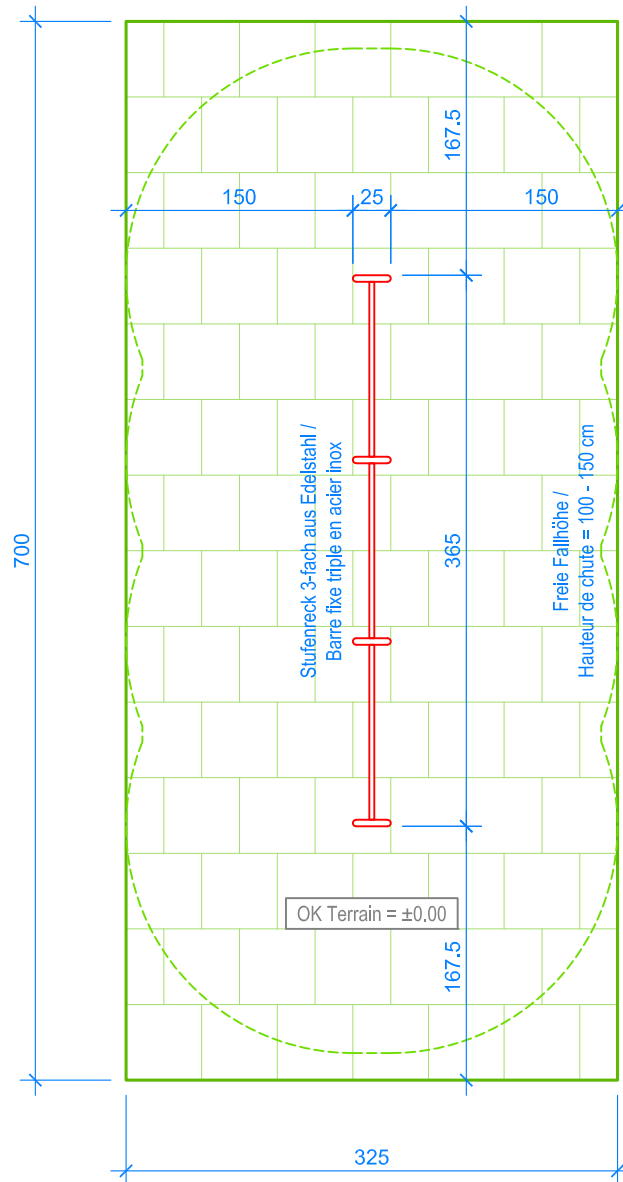
GRUNDRISS / PLAN 1:50
