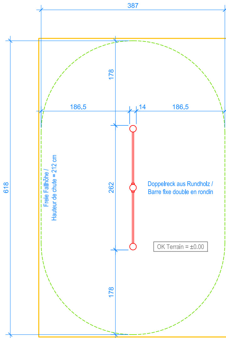
GRUNDRISS / PLAN 1:50
