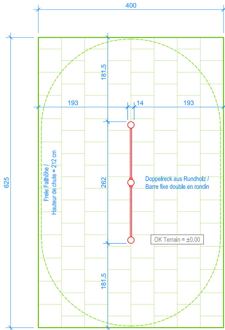
GRUNDRISS / PLAN 1:50
