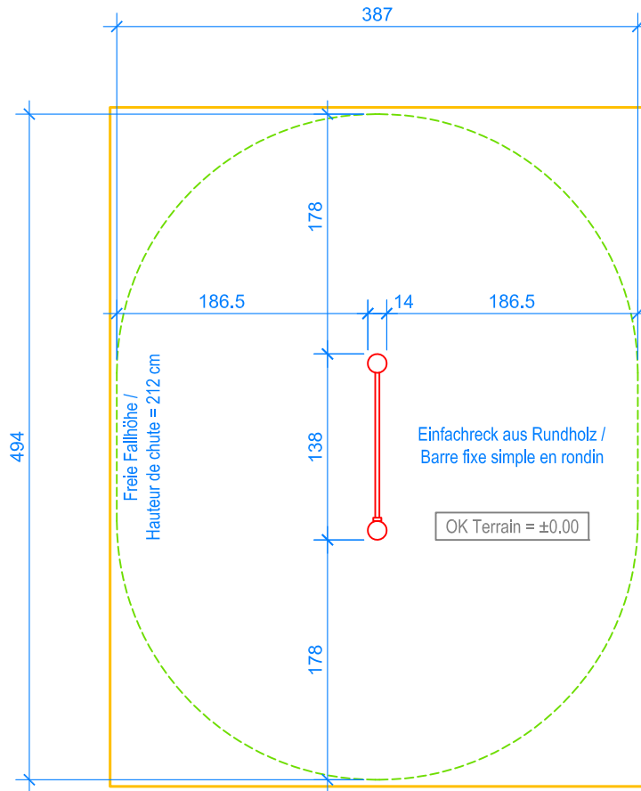
GRUNDRISS / PLAN 1:50
