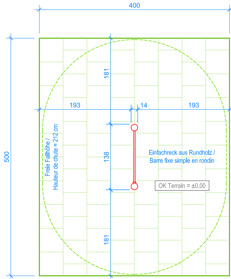
GRUNDRISS / PLAN 1:50
