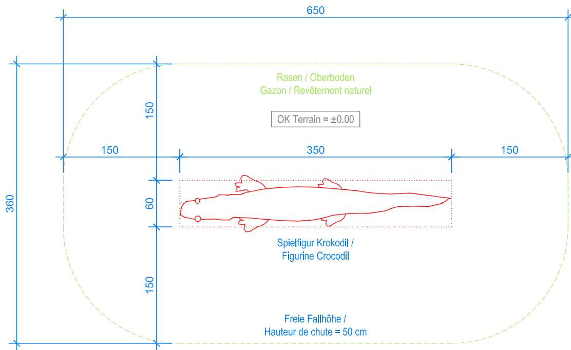
GRUNDRISS / PLAN 1:50
