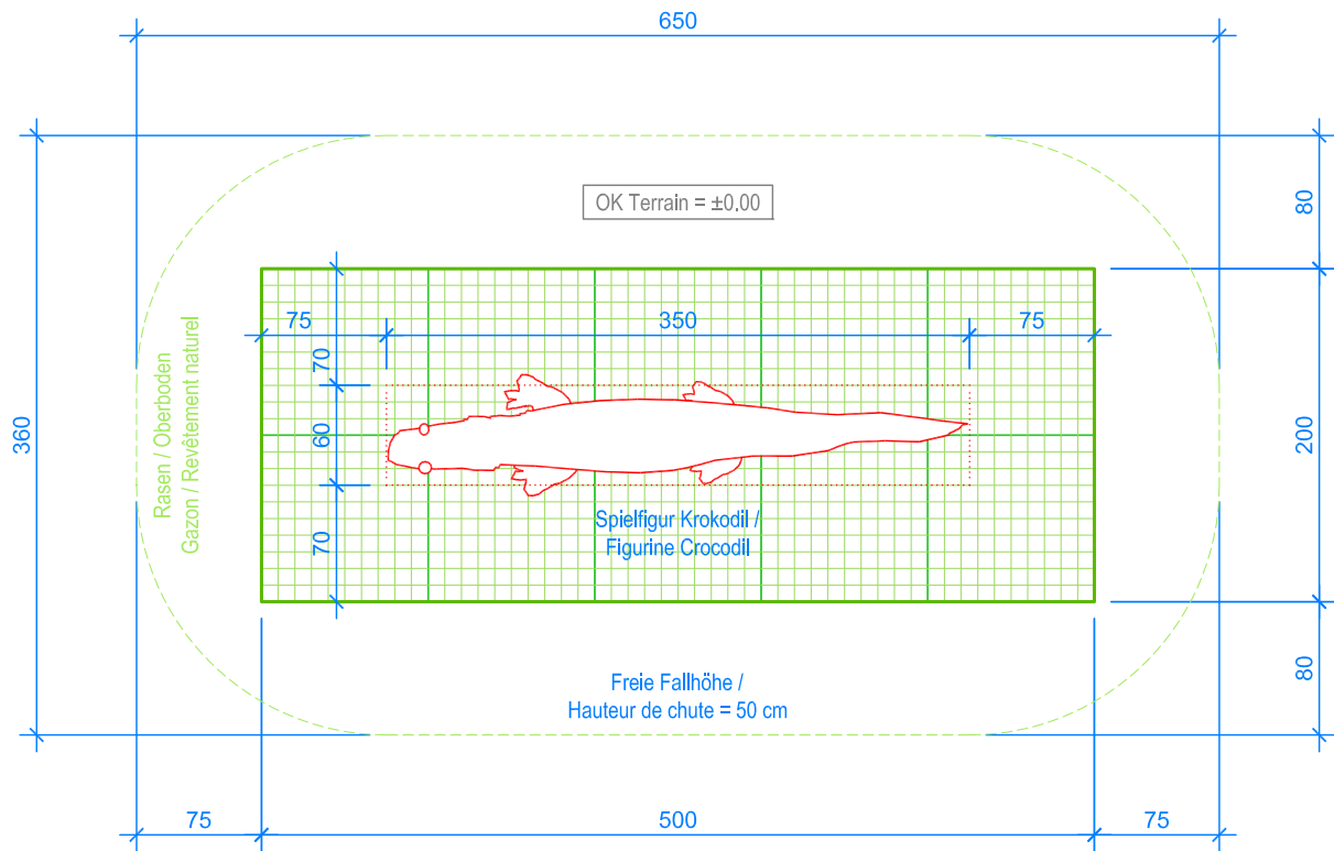
GRUNDRISS / PLAN 1:50
