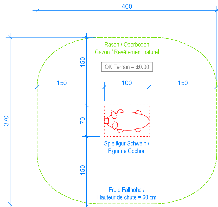
GRUNDRISS / PLAN 1:50
