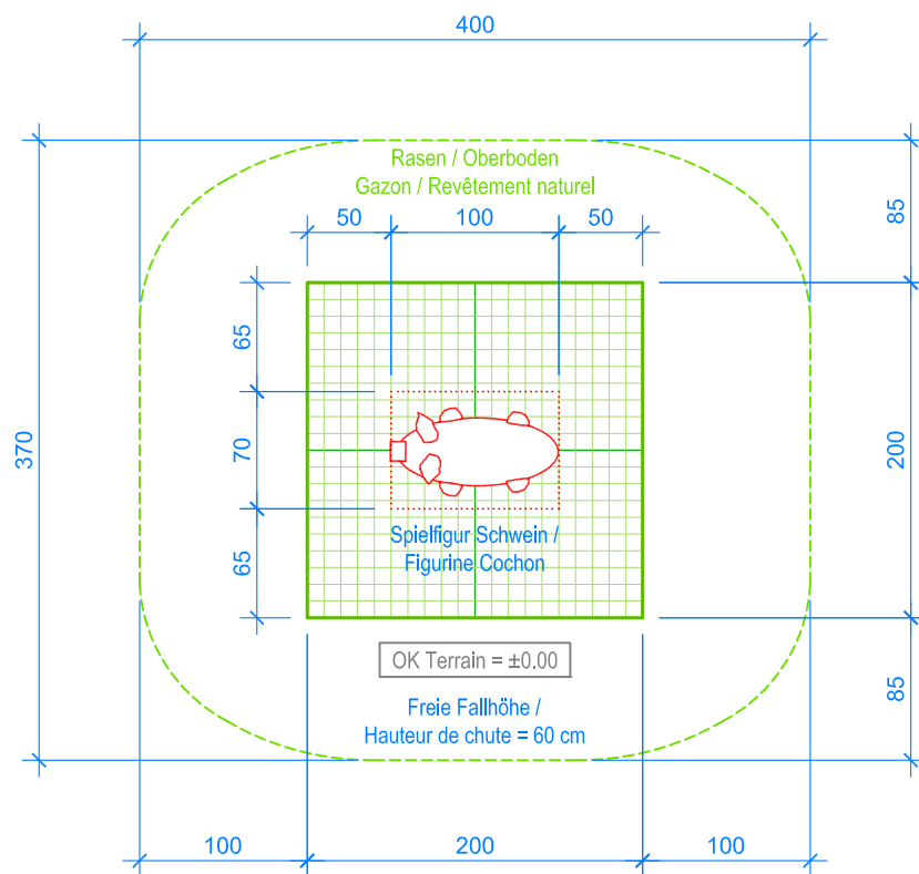
GRUNDRISS / PLAN 1:50
