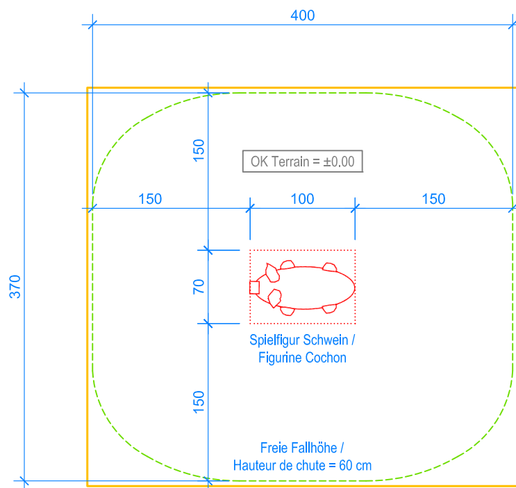
GRUNDRISS / PLAN 1:50
