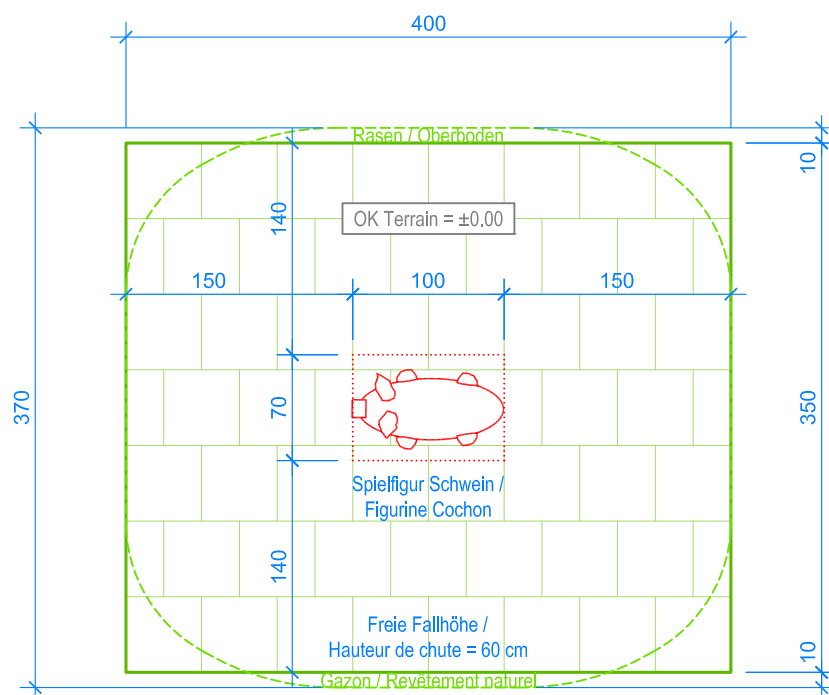
GRUNDRISS / PLAN 1:50
