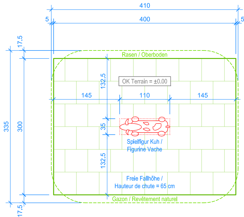
GRUNDRISS / PLAN 1:50
