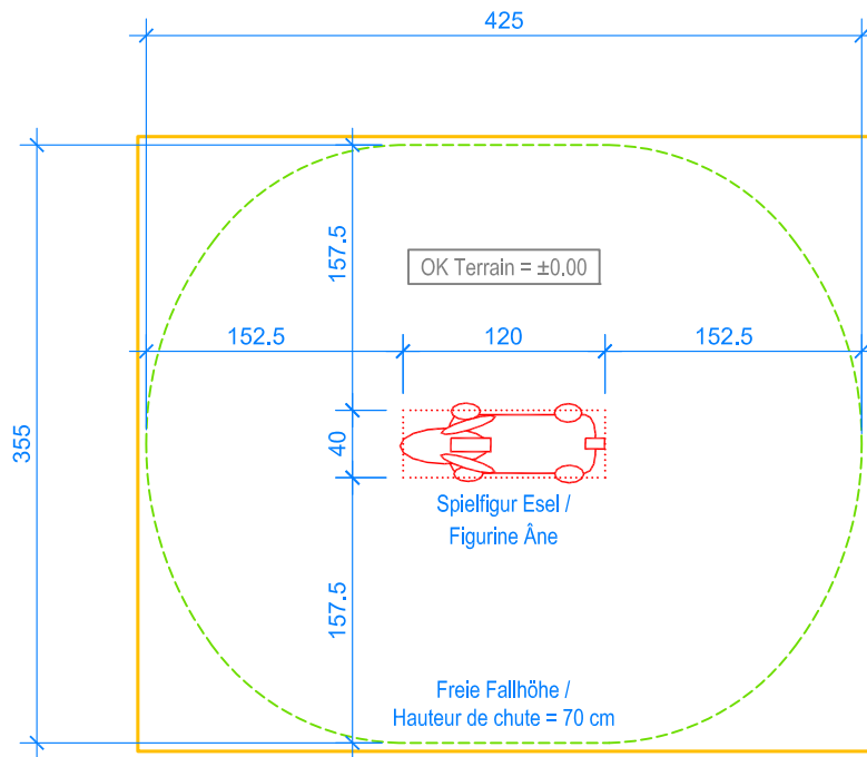
GRUNDRISS / PLAN 1:50
