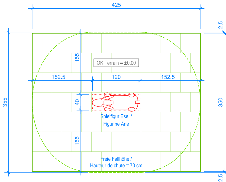
GRUNDRISS / PLAN 1:50
