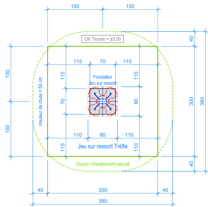
PLAN 1:50
