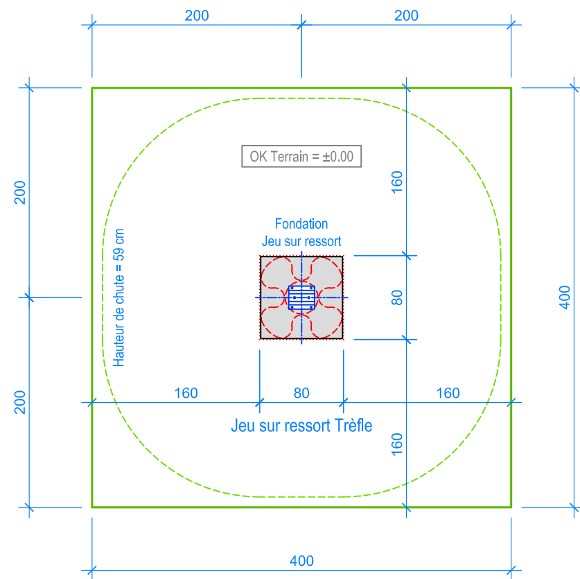
PLAN 1:50
