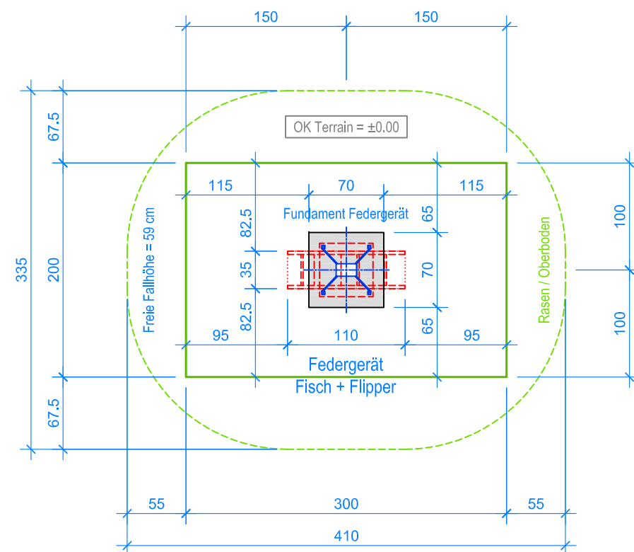
GRUNDRISS 1:50
