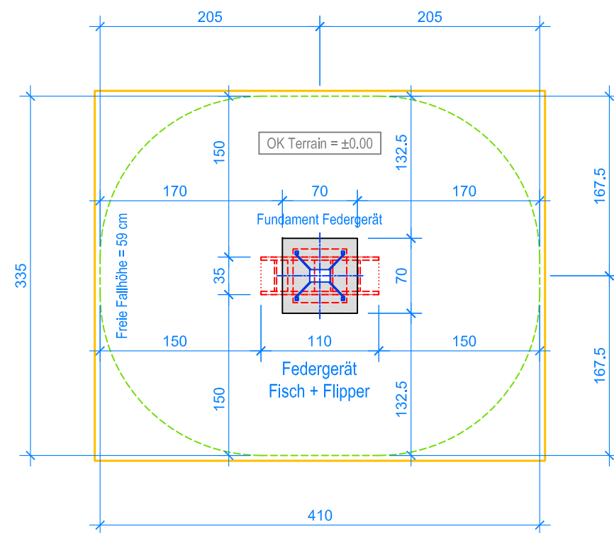
GRUNDRISS 1:50
