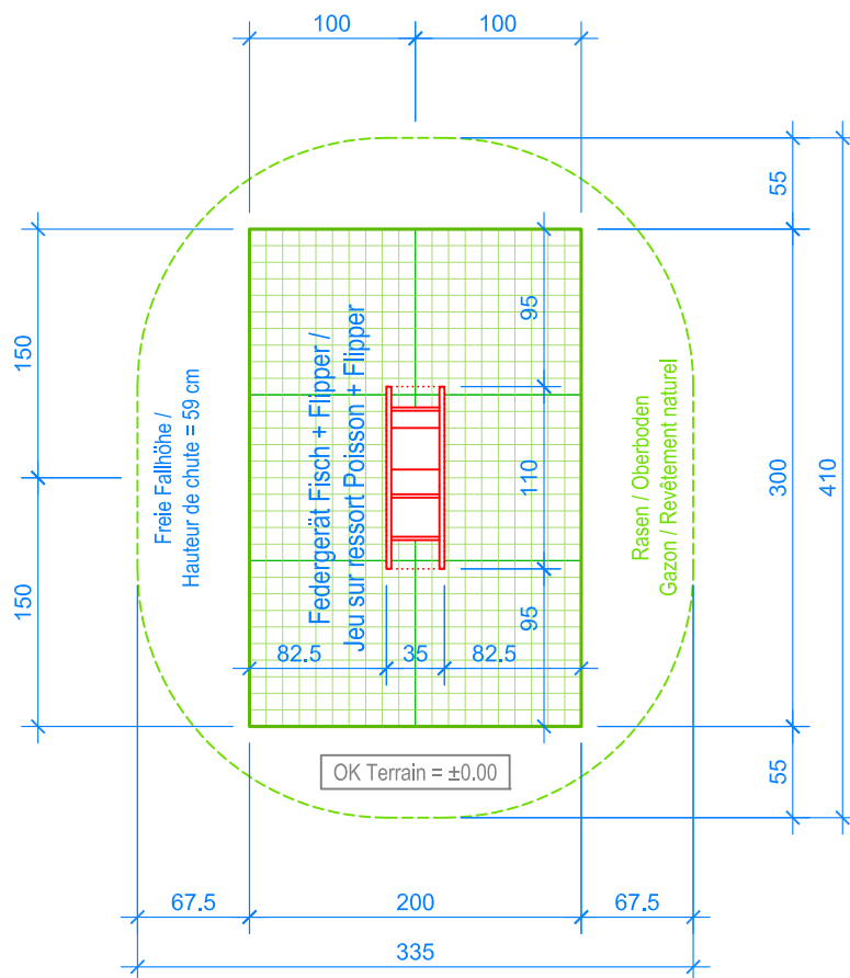
GRUNDRISS / PLAN 1:50
