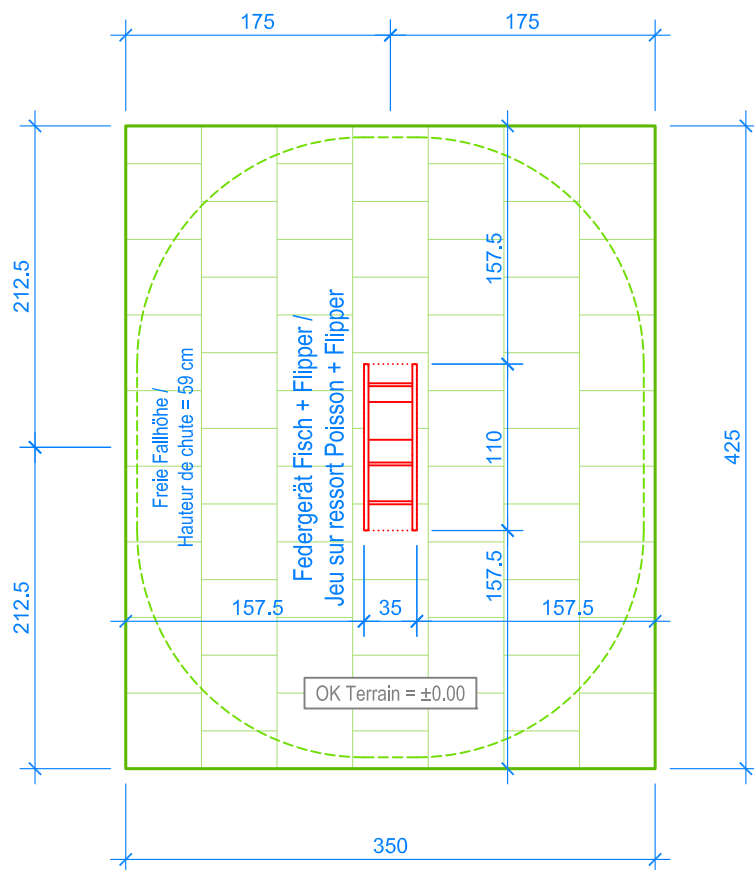
GRUNDRISS / PLAN 1:50
