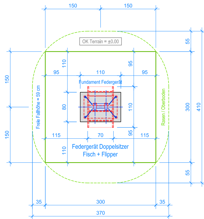
GRUNDRISS 1:50
