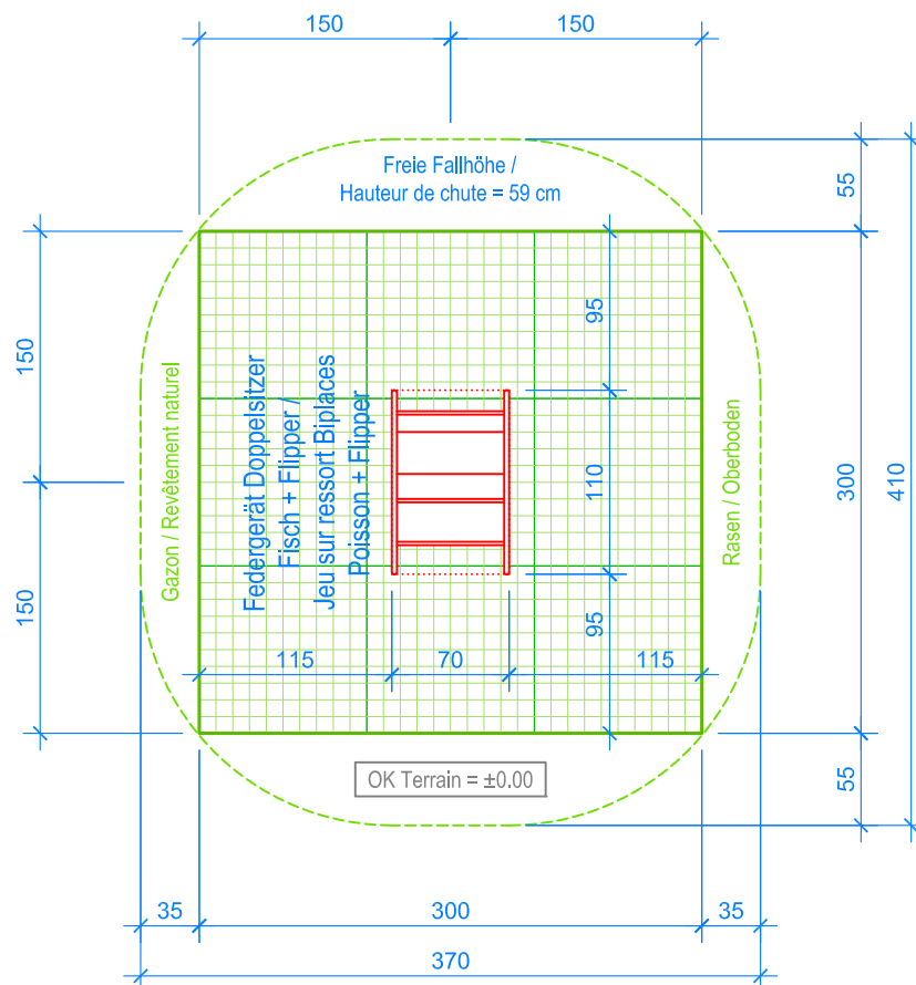
GRUNDRISS / PLAN 1:50
