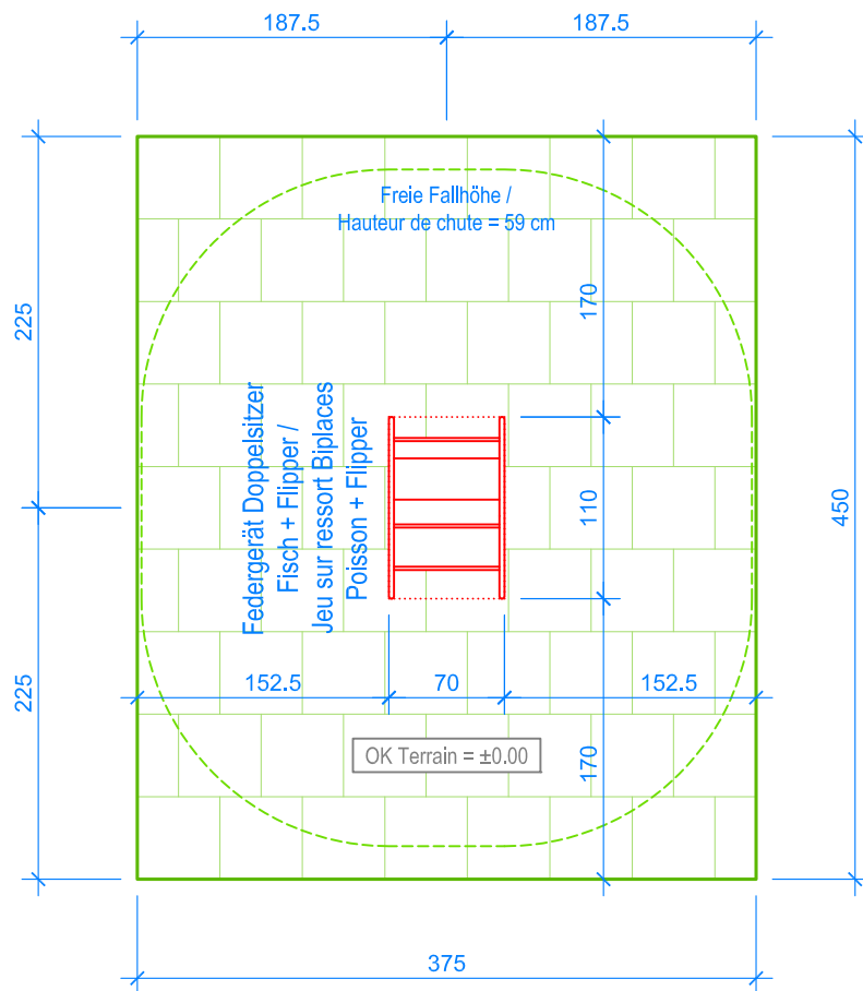
GRUNDRISS / PLAN 1:50
