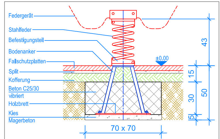
SCHNITT 1:20 FUNDAMENT FEDERGERÄT
