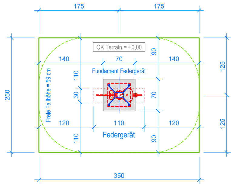
GRUNDRISS 1:50
