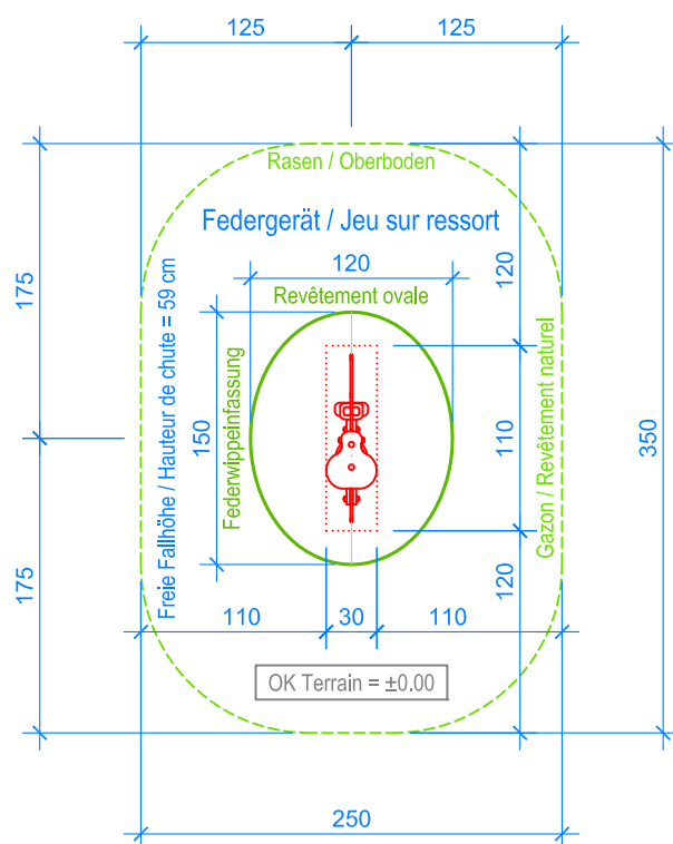
GRUNDRISS / PLAN 1:50
