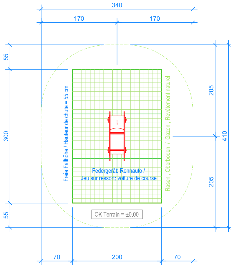
GRUNDRISS / PLAN 1:50
