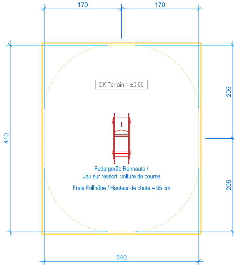
GRUNDRISS / PLAN 1:50
