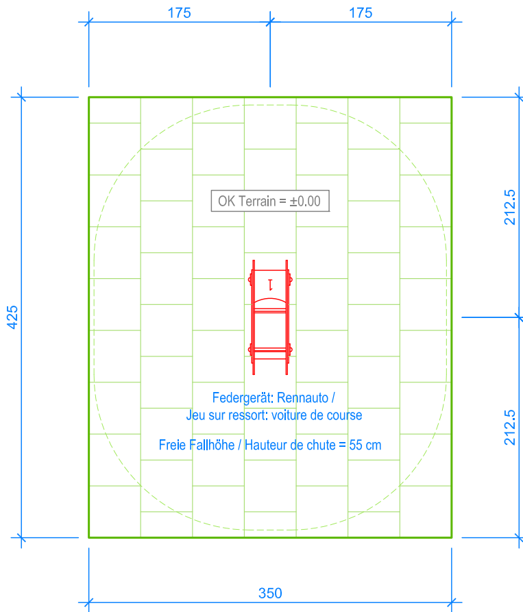
GRUNDRISS / PLAN 1:50
