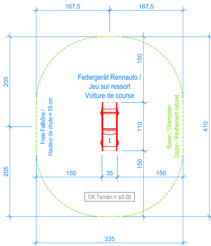
GRUNDRISS / PLAN 1:50
