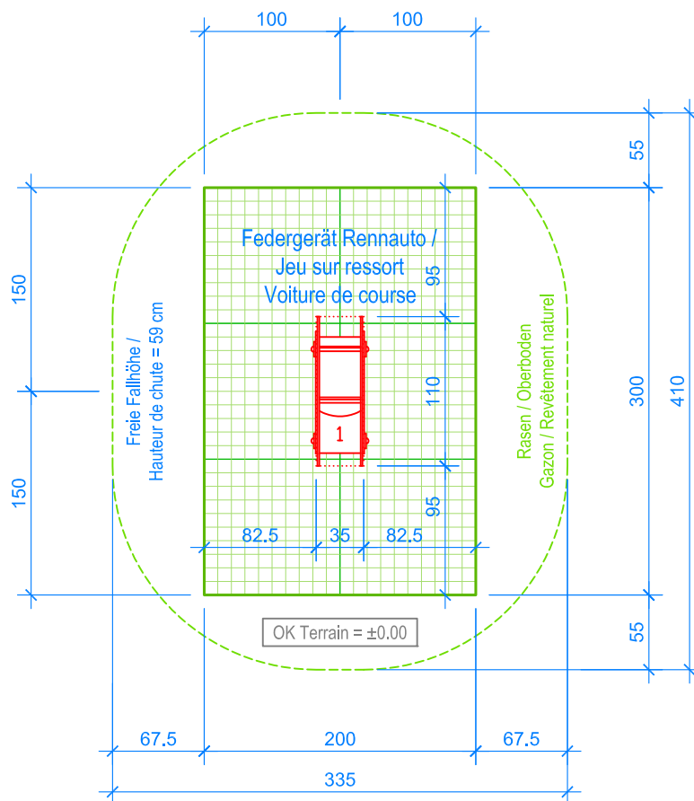
GRUNDRISS / PLAN 1:50
