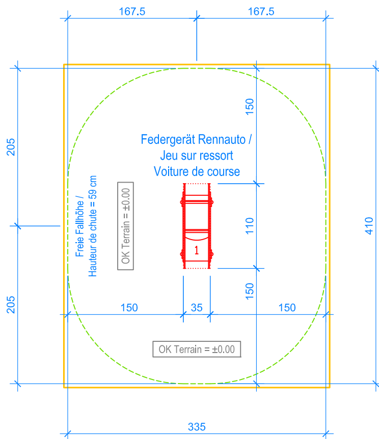
GRUNDRISS / PLAN 1:50
