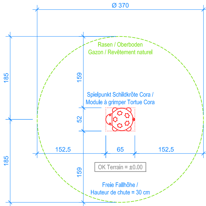
GRUNDRISS / PLAN 1:50
