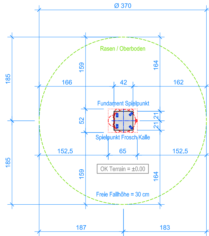
GRUNDRISS 1:50
