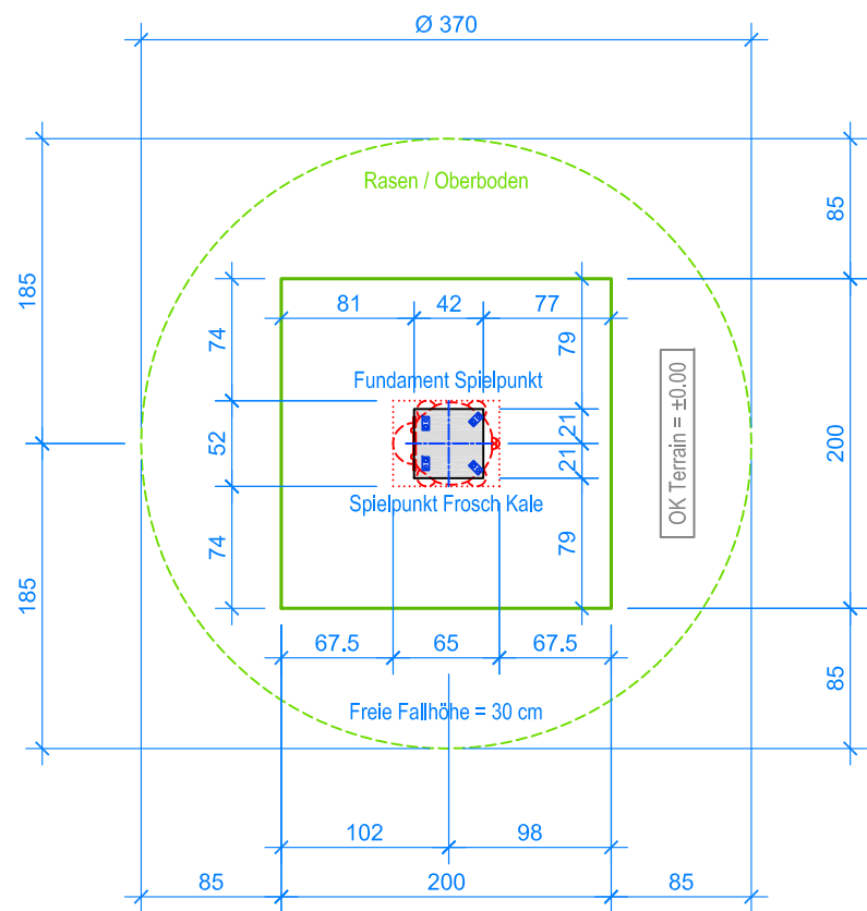
GRUNDRISS 1:50
