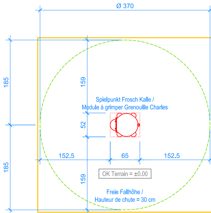
GRUNDRISS / PLAN 1:50
