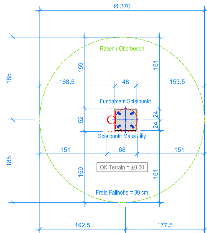
GRUNDRISS 1:50
