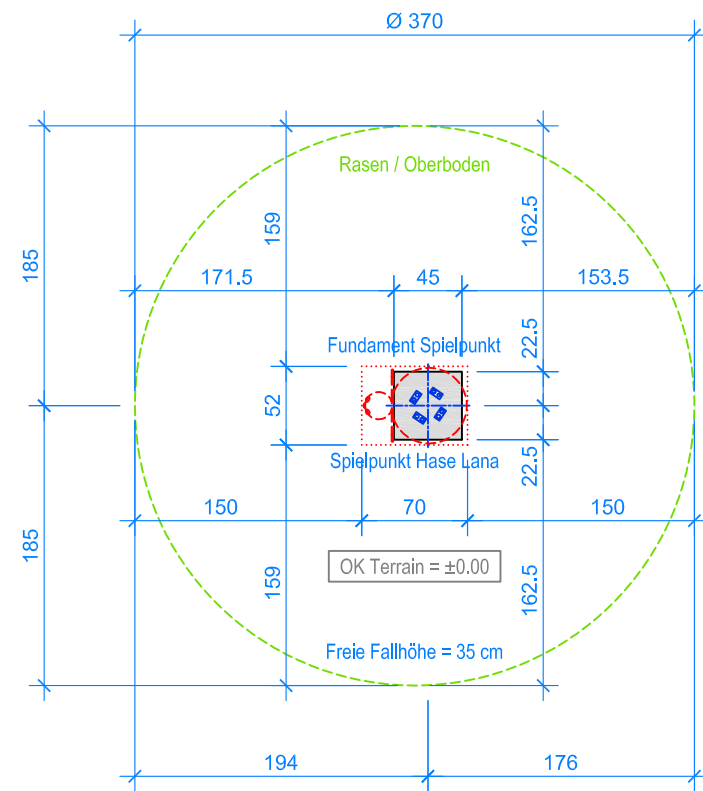
GRUNDRISS 1:50
