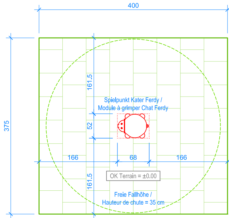
GRUNDRISS / PLAN 1:50
